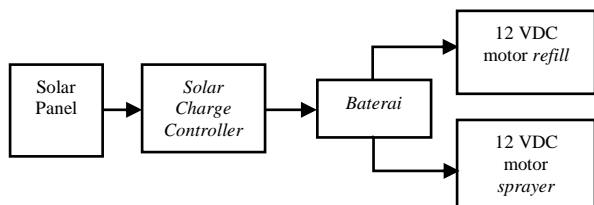
Gambar 6. Diagram blok sistem alat penyemprot pestisida tenaga surya
