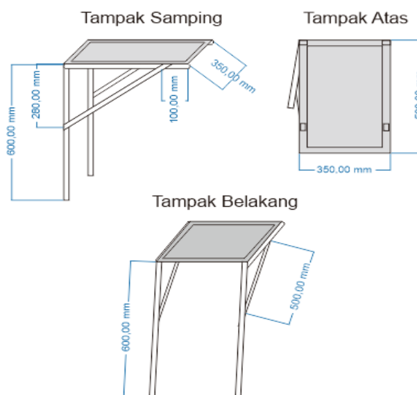
Gambar 8. Desain rangka penyangga panel surya
