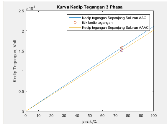
Gambar 6. Kurva Kedip Tegangan Dititik 75% Sepanjang Saluran
