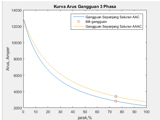
Gambar 4. Kurva Gangguan Hubung Singkat Tiga Fasa Dititik Gangguan 75% Sepanjang Saluran
