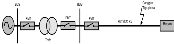
Gambar 1. SingleLine Gangguan Satu Fasa Ke Tanah Pada Sisi Penyulang
