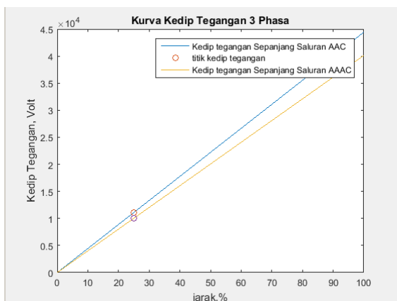
Gambar 5. Kurva Kedip Tegangan Dititik 25% Sepanjang Saluran
