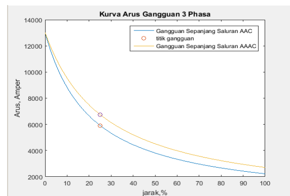
Gambar 3. Kurva Gangguan Hubung Singkat Tiga Fasa Dititik Gangguan 25% Sepanjang Saluran
